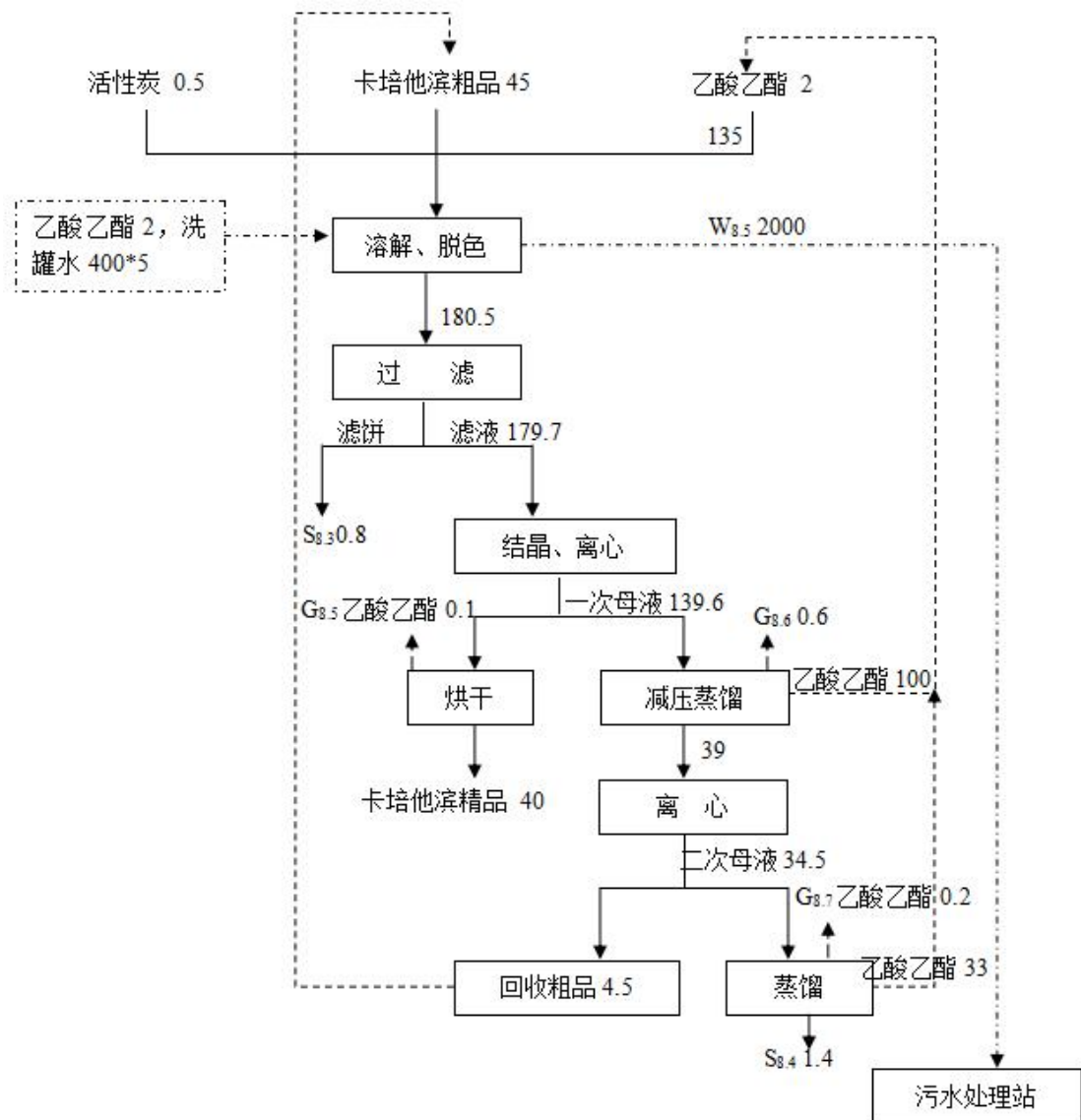
2.2-10 卡培他滨精制工艺流程图
