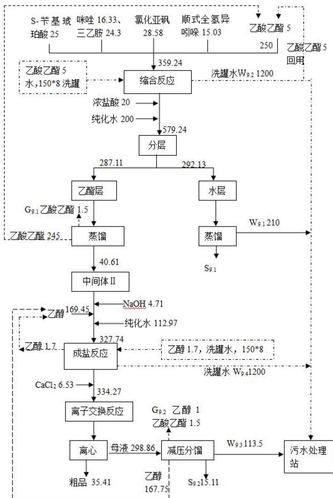
2.2-11 米格列奈钙粗品工艺流程图
