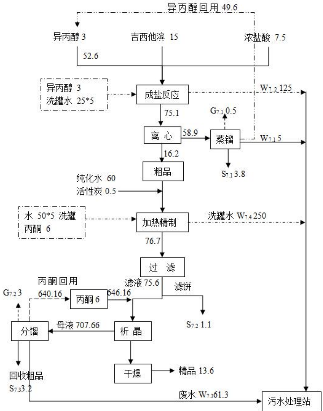
2.2-8 盐酸吉西他滨工艺流程图
