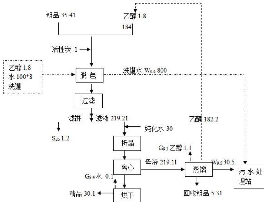
2.2-12 米格列奈钙精制工艺流程图
