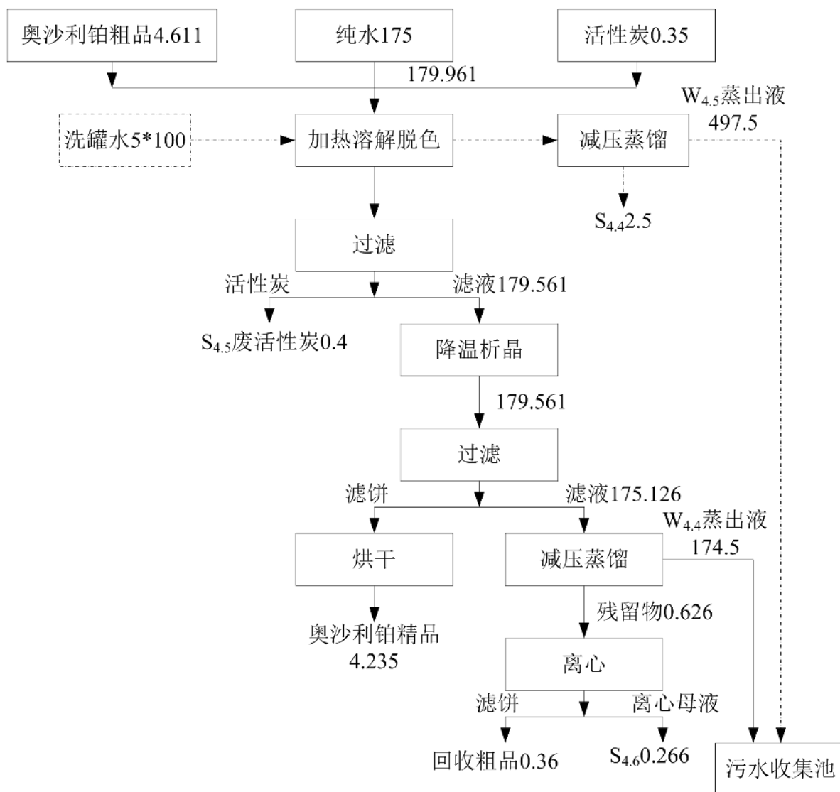
图 2.2-5 奥沙利铂精制工艺流程
