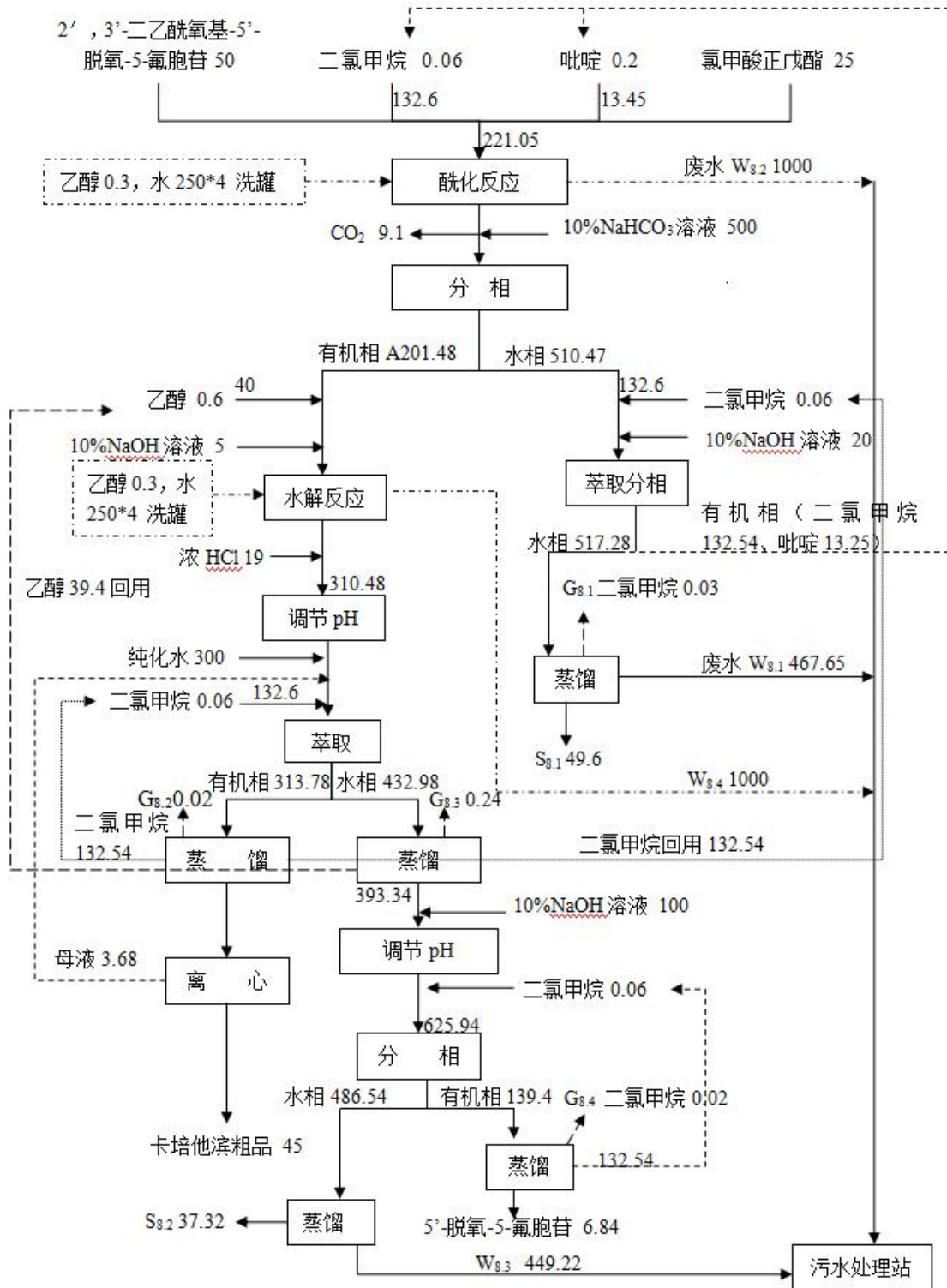
2.2-9 卡培他滨粗品工艺流程图
